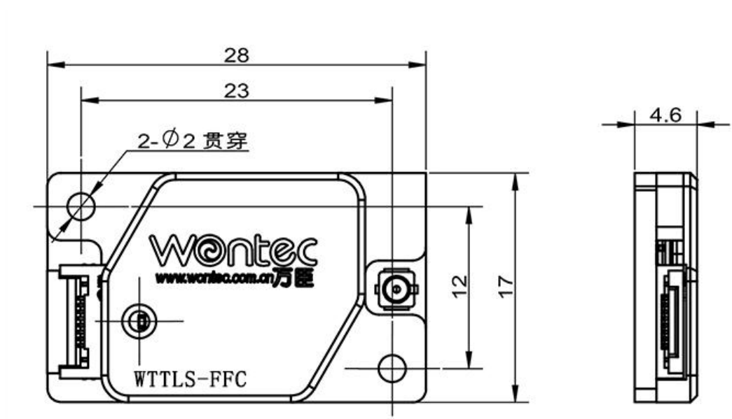
WTLLS-FFC 尺寸图:
