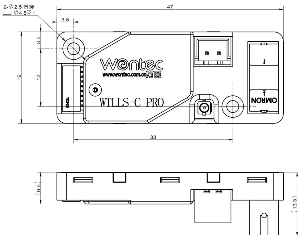
WTLLS-C PRO 尺寸图:
