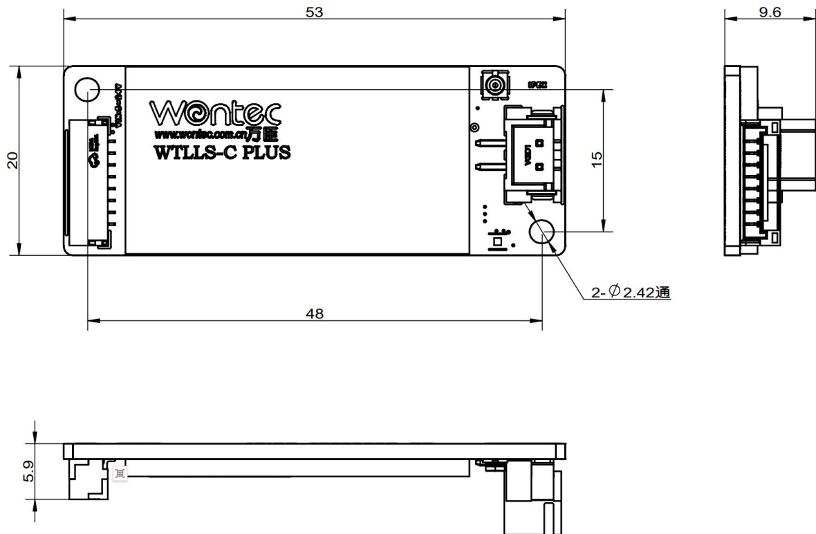
WTLLS-C PLUS 尺寸图:
