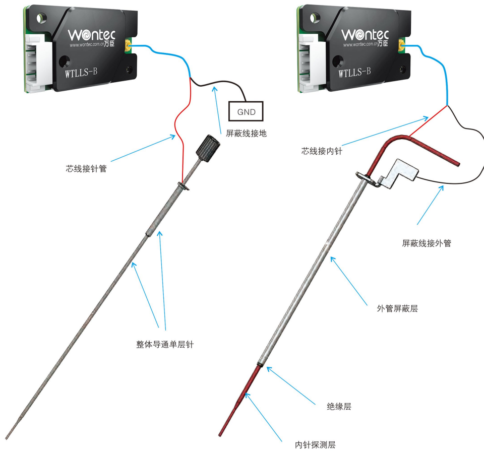
单层针接线示意图
