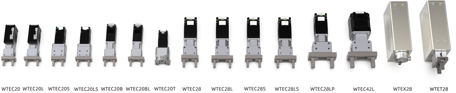
各型号电动夹爪尺寸对比
