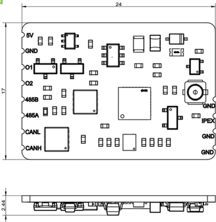
反馈型液面传感器 贴片C型 ·反馈型电容式液面探测，闭环控制更可靠。
