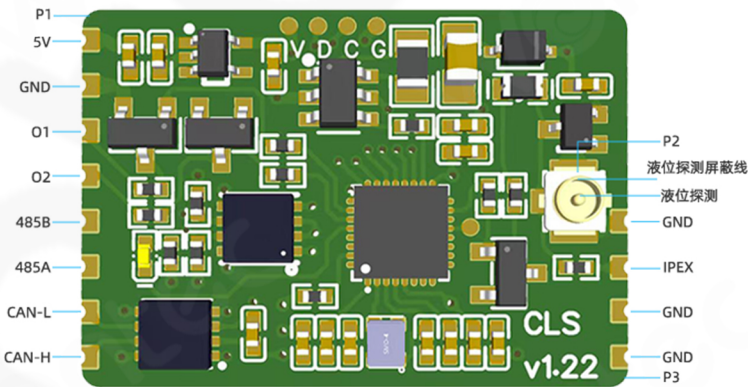
电路接线完成后，上电后LED指示灯快速闪烁一次，证明接线正确。 当检测到液面时候，指示灯快速闪烁一次，表示探测液位成功。
