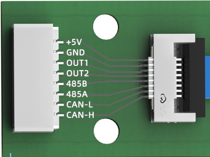
转接板
